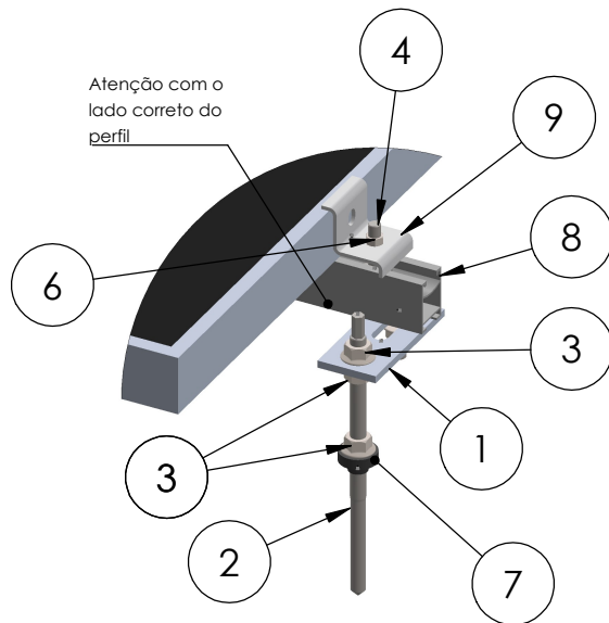
DETALHE A ESCALA 1 : 5
